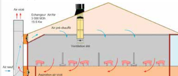
ECHANGEUR D'AIR EXTÉRIEUR
