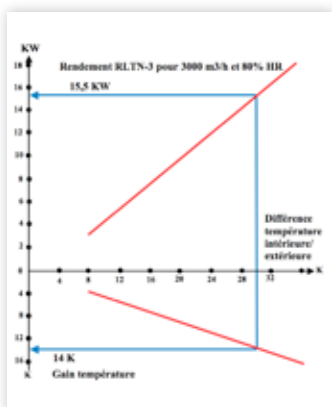
ECHANGEUR D'AIR EXTÉRIEUR
