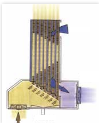
ECHANGEUR D'AIR COMBLE
