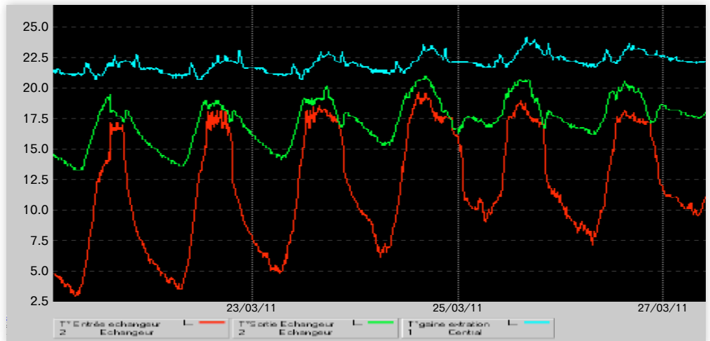
ECHANGEUR D'AIR COMBLE
